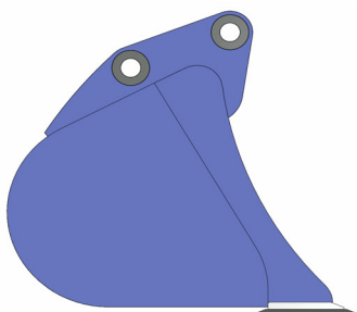
PROFIL GR-CS-S STD/R* (standard/wzmocniona) koparki 35-50t
