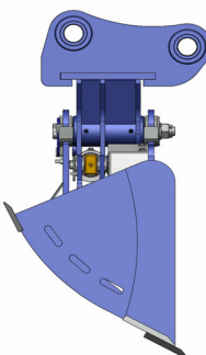
PROFIL 700-U STD/R* (standard/wzmocniona) koparki 19-30t
