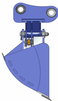
PROFIL 900-U STD/R* (standard/wzmocniona) koparki 24-42t
