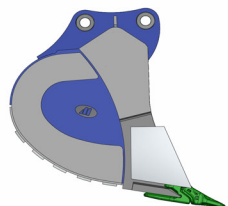
PROFIL 30T HD**** koparki 32-39t lemesz 410x60mm
