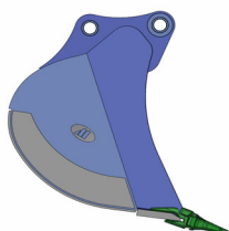
PROFIL 140 STD/R* koparki 30-38t lemiész 350x50mm
