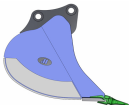
PROFIL 130 STD/R* koparki 26-33t lemiész 300x45mm
