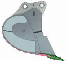
PROFIL 40T HD**** koparki 39-47t lemesz 440x60mm
