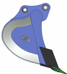
PROFIL 110 HD**** koparki 13-17t lemięsz 300x30mm
