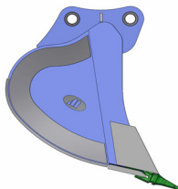
PROFIL 125 HD**** koparki 21-26t lemesz 300x40mm
