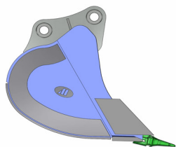
PROFIL 130 HD**** koparki 26-33t lemiész 300x45mm
