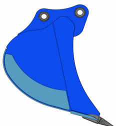
PROFIL 110 STD/R* koparki 13-17t lemięsz 300x30mm
