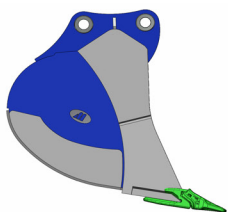
PROFIL 30T STD/R* koparki 32-39t lemesz 410x50mm
