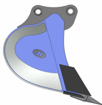
PROFIL 120 HD**** koparki 17-21t lemesz 300x35mm
